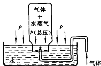
图 1-1 用排水取气法收集气体
