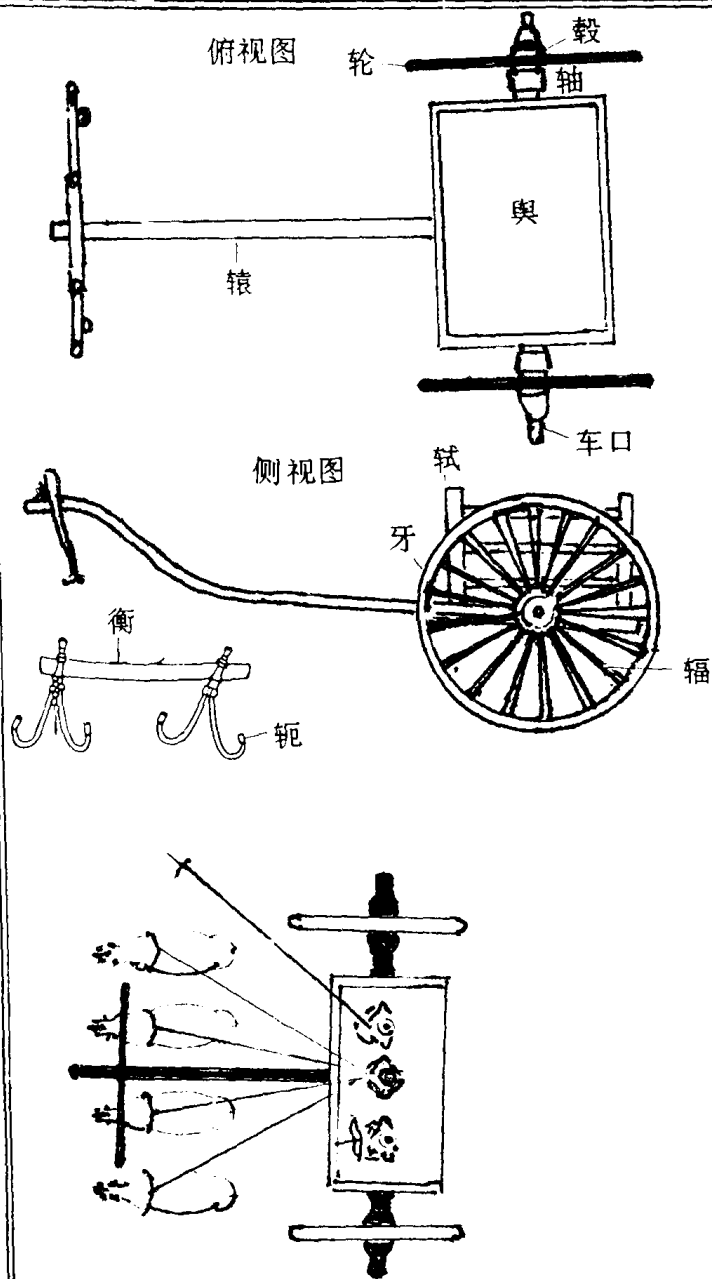
兵图九：战车
