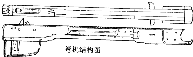
战国弩机结构发射示意图
