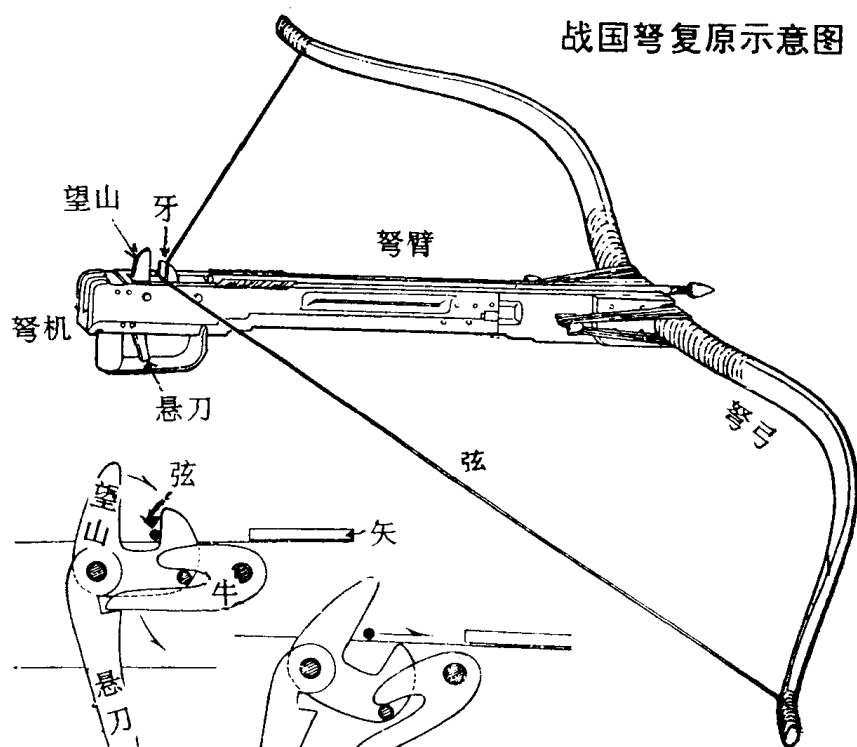
战国弩机结构发射示意图
