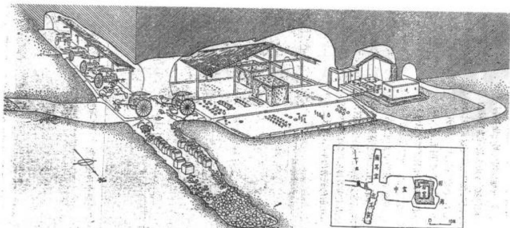
▲图①满城刘胜墓 复原图
