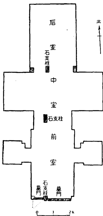
插圖三 睢寧九女墩漢墓平面圖
