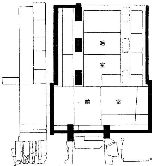
插圖四 銅山縣苗山漢墓平面(右)、剖面圖(左)
