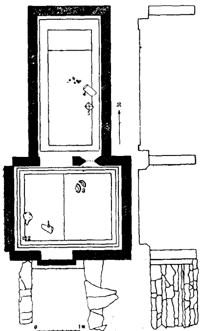
插圖五 銅山縣周莊漢墓平面 (左)、剖面圖(右)
