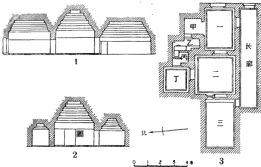
插圖二 徐州市茅村漢墓平面、斷面圖
