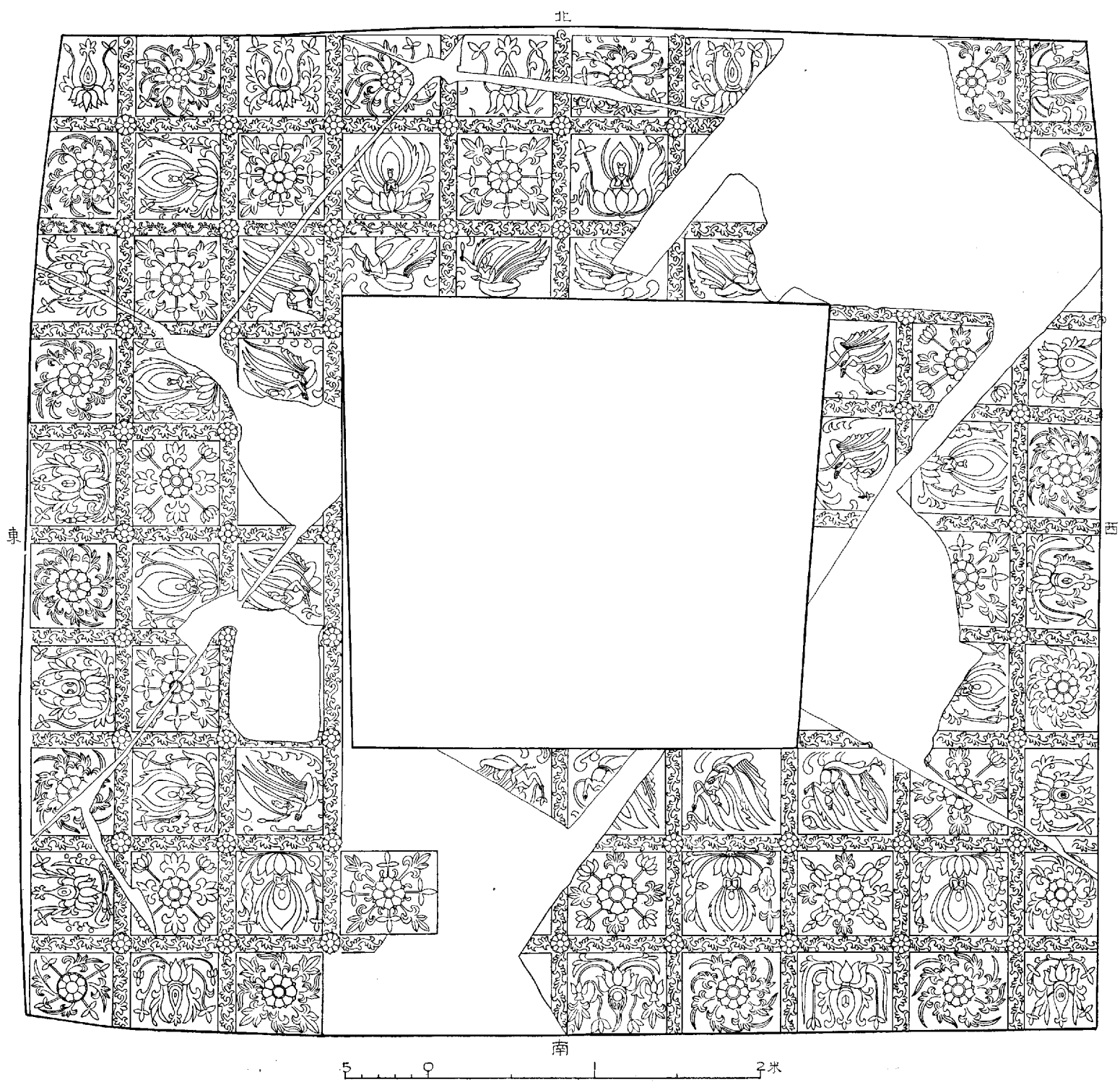
第一窟平基圖
