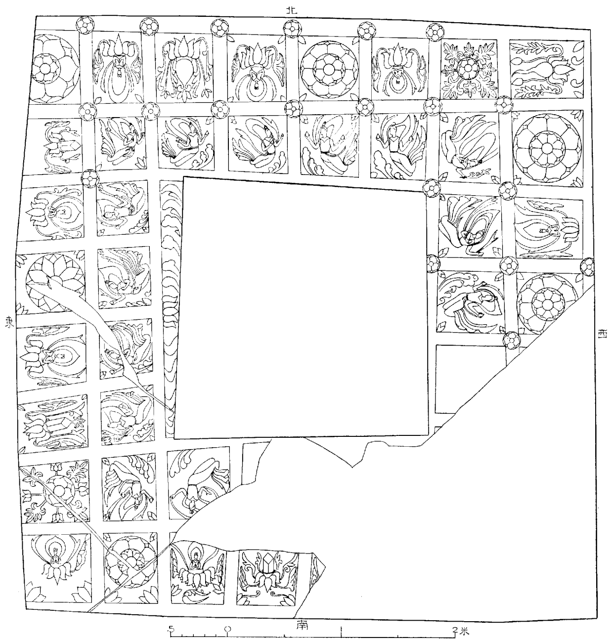
第三窟平基圖
