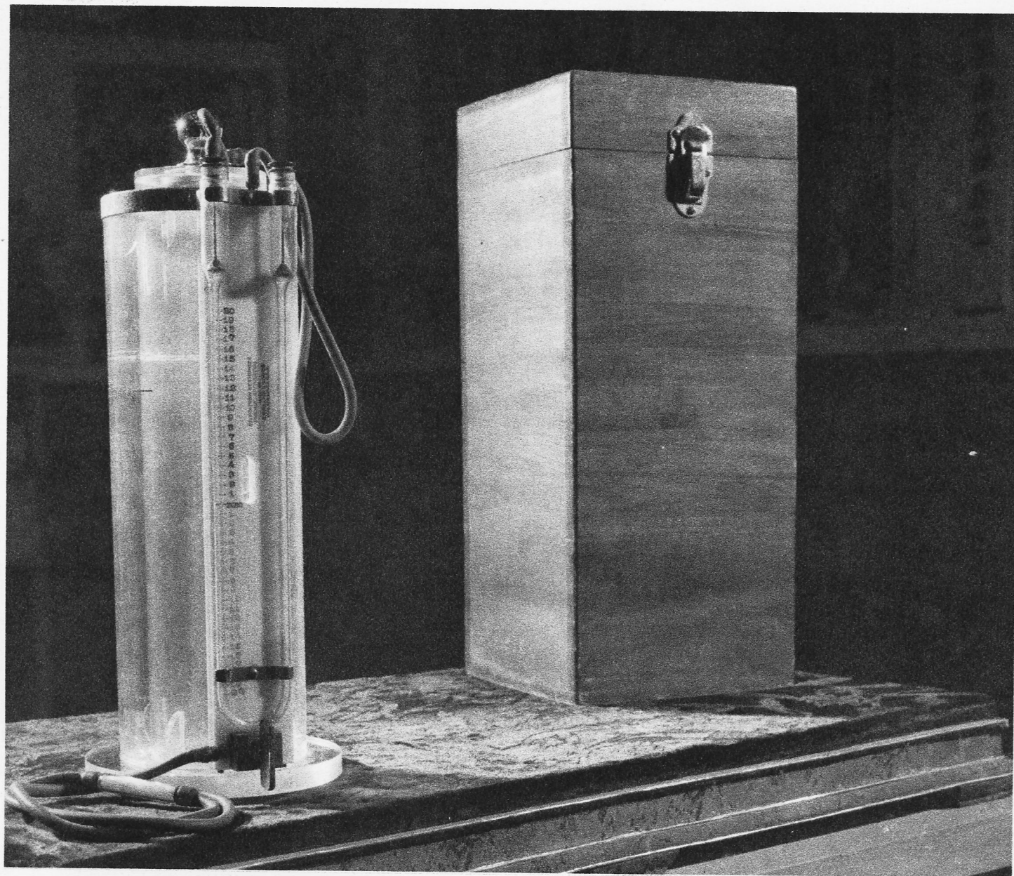
这是白求恩同志发明的人工气胸器
