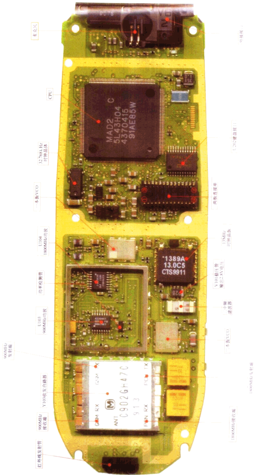
诺基亚6150手机元件实物图A面
