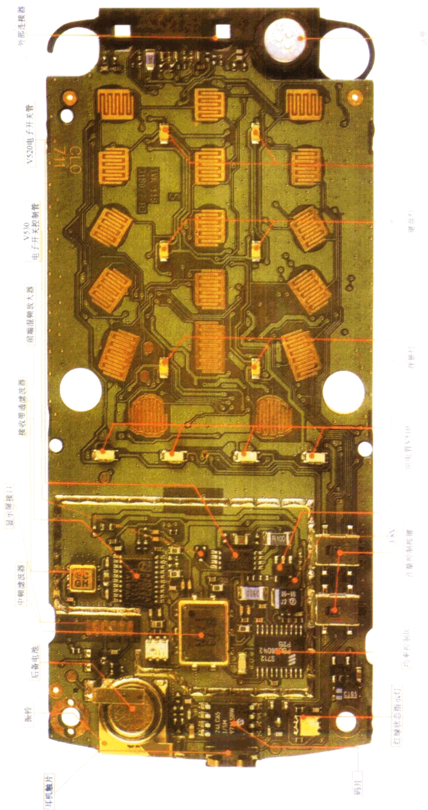
爱立信788 (768) 手机元件实物图B面
