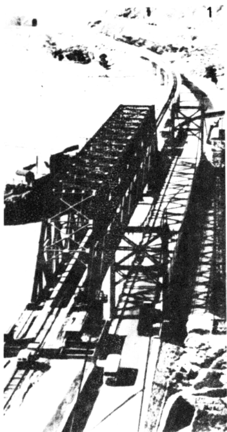
1、河津龙门铁路、公路大桥
