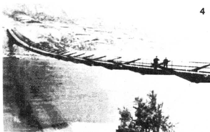
4、平陆南沟黄河大吊桥
