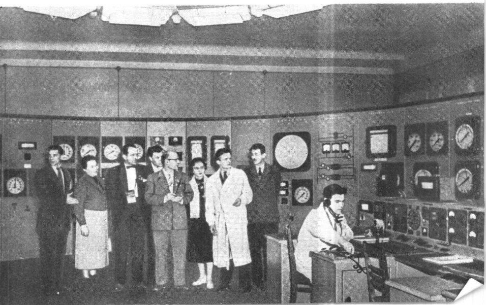
外賓們參觀苏联原子能發電站的中央操縱台。
