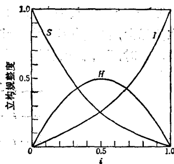
图 1.1 Bovey 模型
