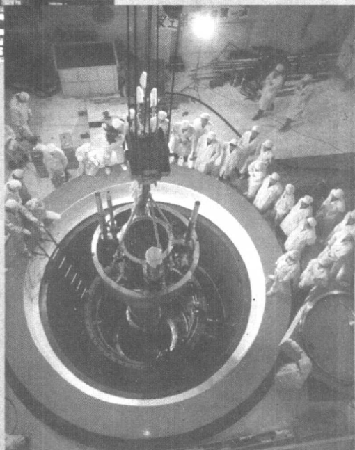
低温核供热反应堆
