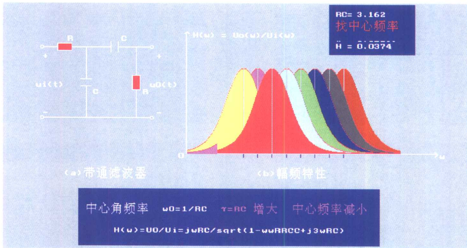
图 8-16 RC 无源带通网络特性的变化规律
