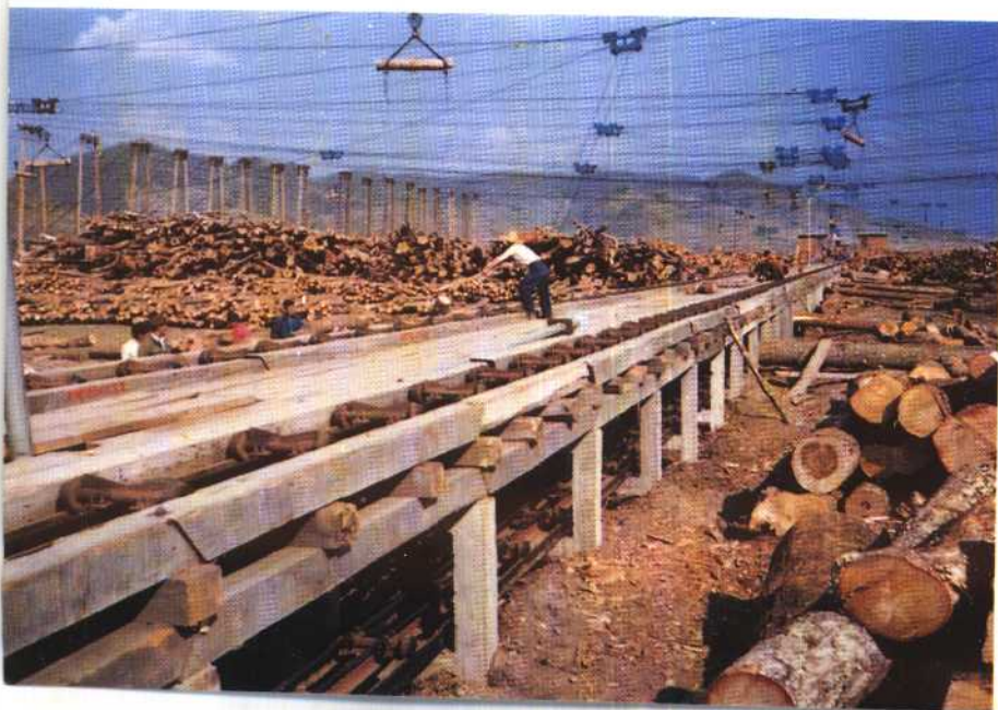
造材归楞
