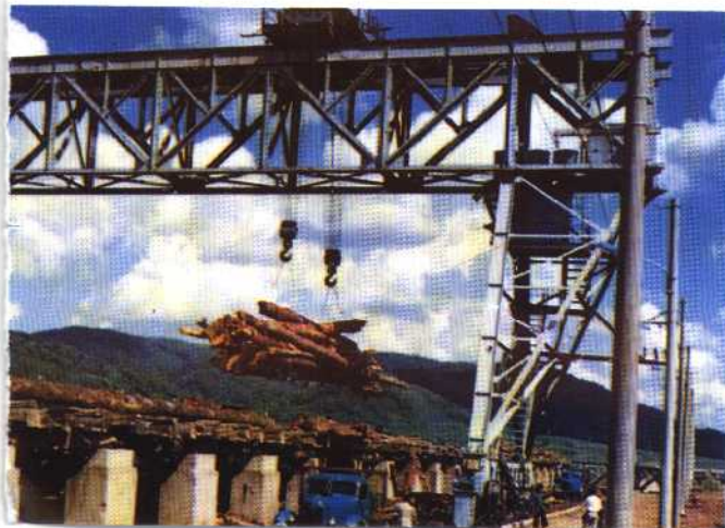
吊材卸车
