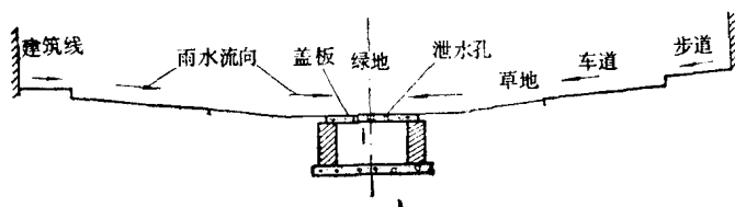
图1-3 地面式暗沟在道路断面内布置示例(二)
