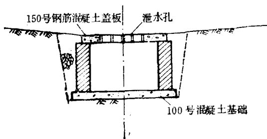
图1-4 地面式暗沟断面做法示意
