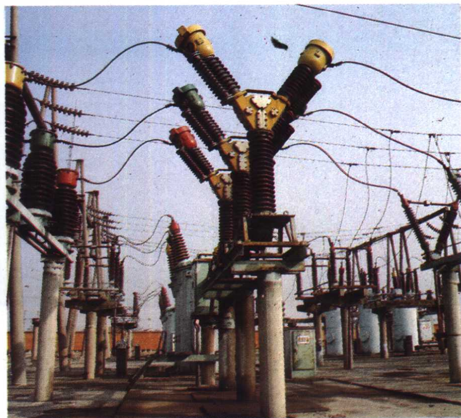
长江埠110千伏变电站
