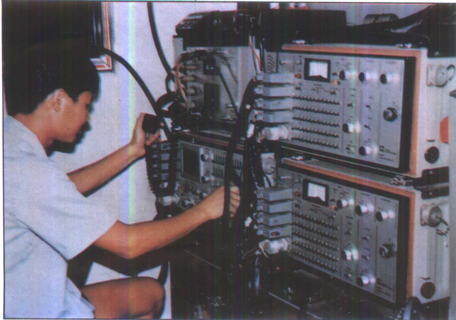
80年代从美国引进的 DFS-V120 道数字地震仪 正在野外施工
