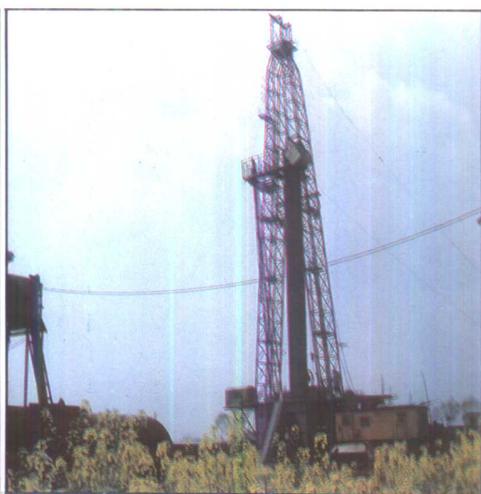
F320-4DH-2 型 6000 米钻机
