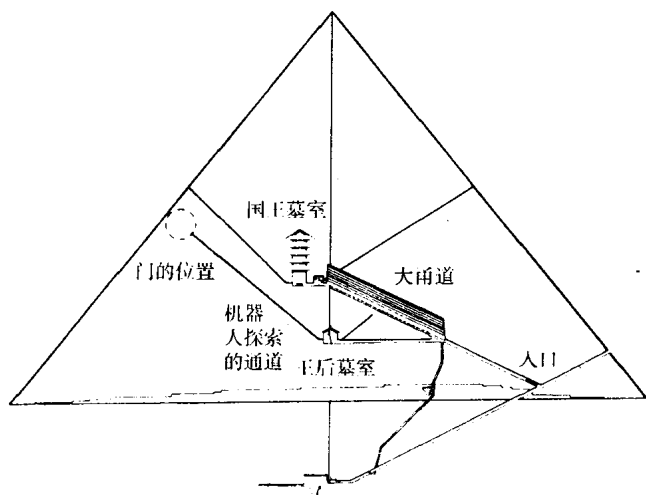
展示墓室、雨道和通道的大金字塔横截面
