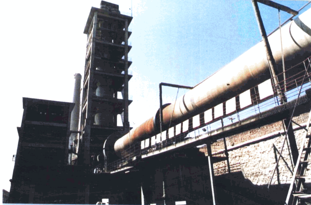
唐山市第一水泥廠回轉窯
