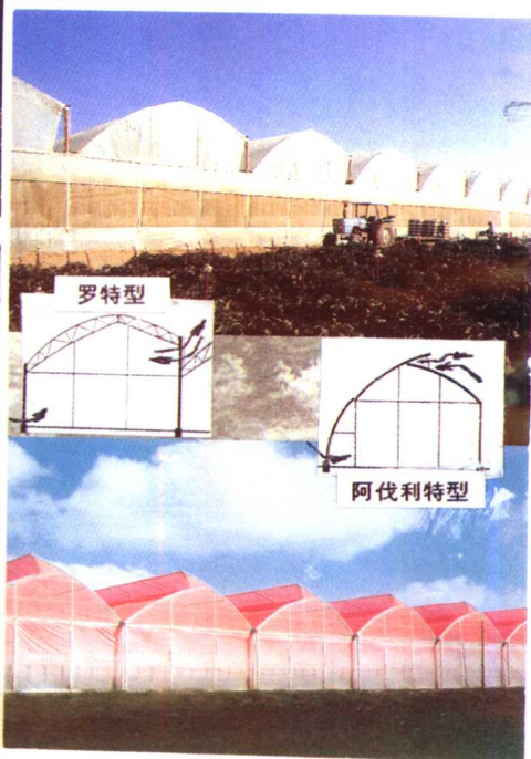
8. 罗特型和阿伐利特型薄膜温室
