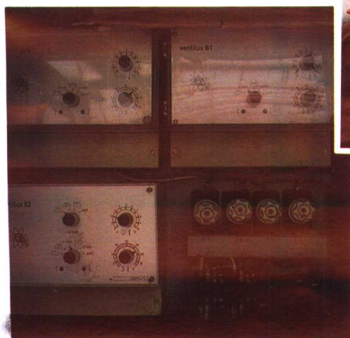
21. 玻璃温室喷灌, 天窗 开启电动控制盘
