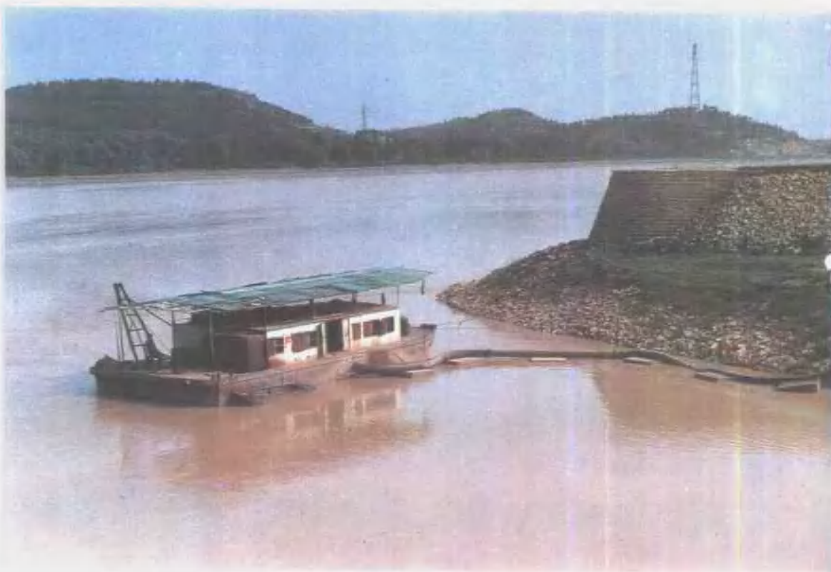
东阿县吸泥船放淤固堤
