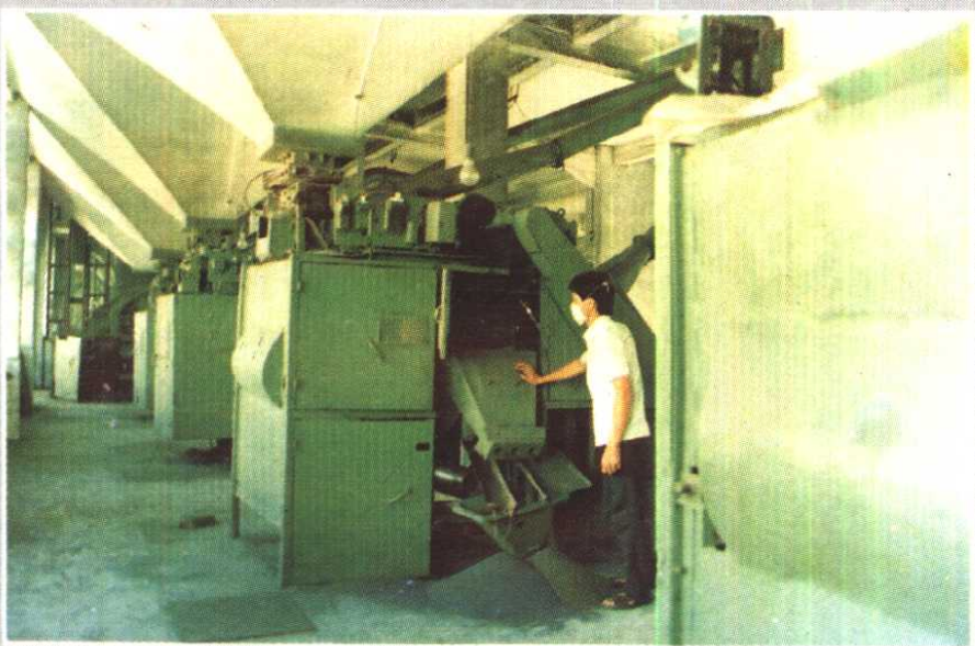
乌场钛矿选矿车间
