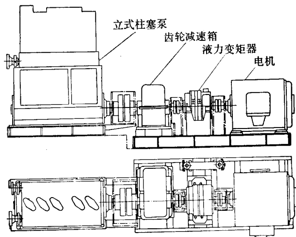
图 6 立式高压甲铵泵外形
