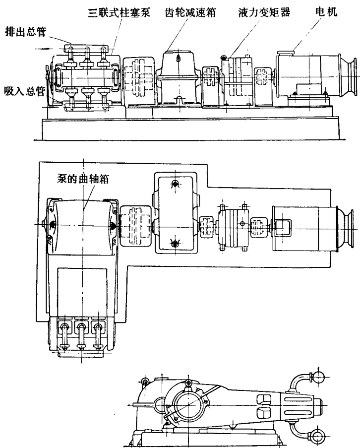
图 1 卧式甲铵泵外形
