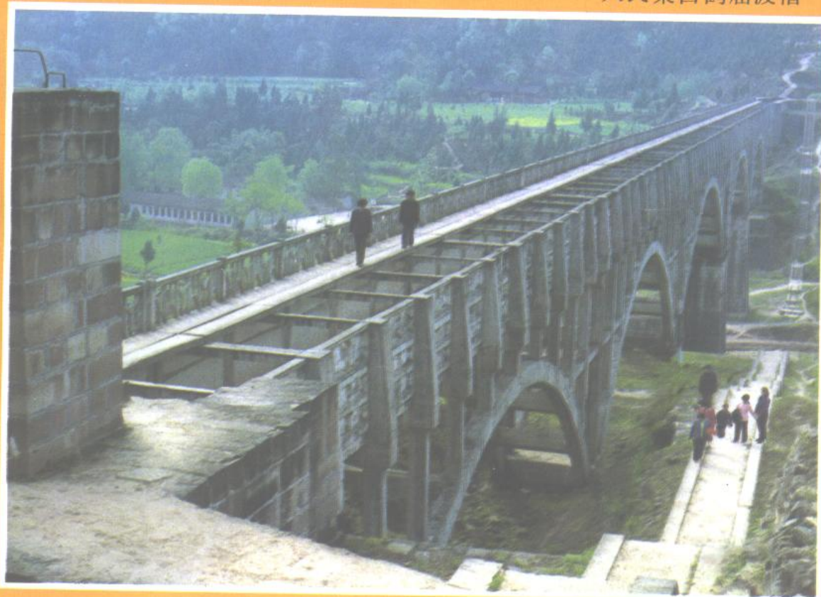
人民渠白鹤庙渡槽
