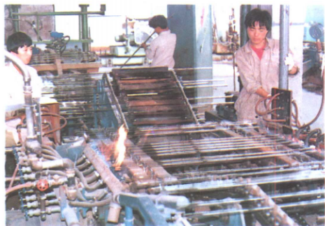
高铅玻璃厂生产车间
