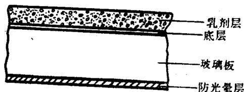
图 1-1 超微粒干版结构
