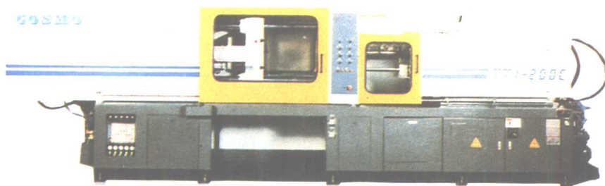
公司下属塑料厂的注塑机
