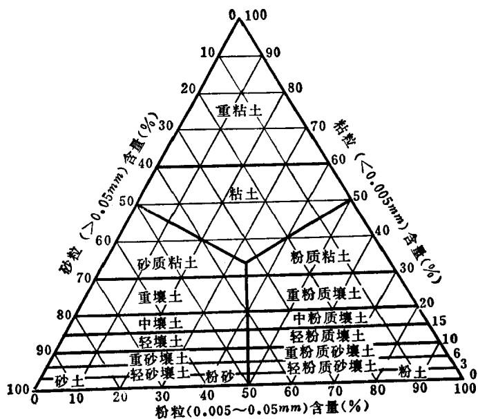
附图 1-1 土 的 分 类
