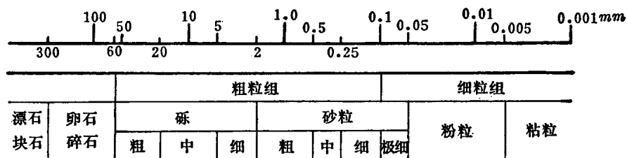
图 1-1 粒组划分图
