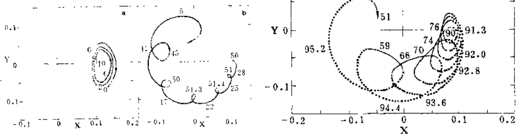
图 5 一个自由边界面和一个刚性边界面情况下,振荡型不稳定模中流体质点的水平投影轨迹
