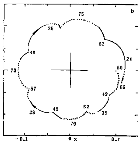
图2 两个自由边界情况下,振荡型不稳定模中流体质点的水平投影轨迹。流体质点的初始高度分别为 (a) z(0)=0.1 , (b) z(0)=0.5 , (c) z(0)=0.9 ( T=10^3 , R=5 \times 10^3 , P=0.025 , a=5.0 )
