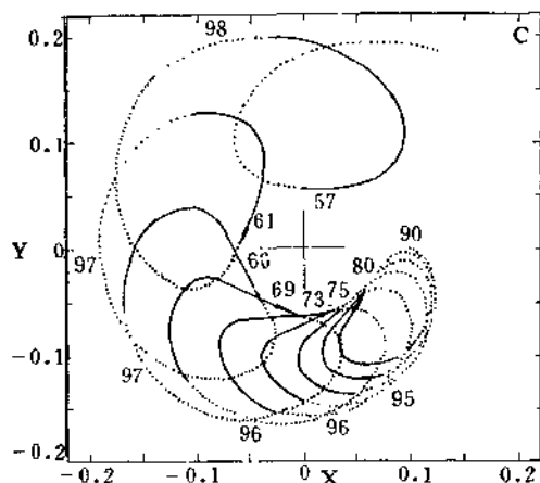
图2 两个自由边界情况下,振荡型不稳定模中流体质点的水平投影轨迹。流体质点的初始高度分别为 (a) z(0)=0.1 , (b) z(0)=0.5 , (c) z(0)=0.9 ( T=10^3 , R=5 \times 10^3 , P=0.025 , a=5.0 )
