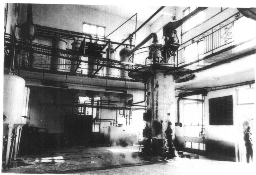
油脂化工厂提炼车间
