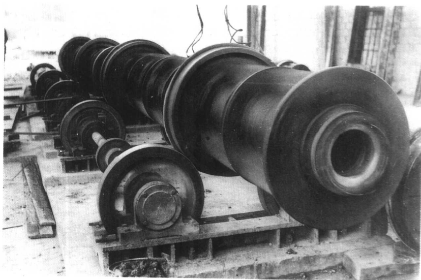
台江县预制厂水泥电杆生产设备
