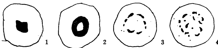
图1 中柱的类型
