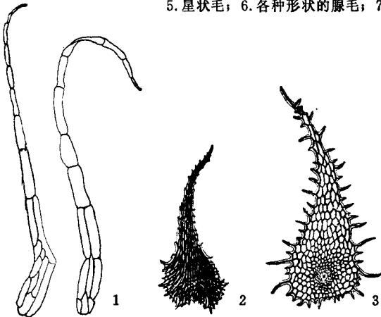
图2 毛的类型
