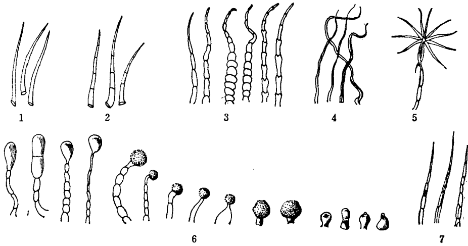
图2 毛的类型
