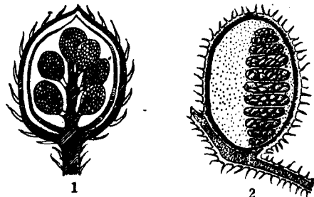
图10 1. 大孢子囊纵剖面；2. 小孢子囊纵剖面。
