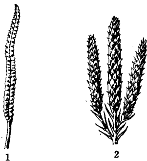
图 11 1. 瓶尔小草孢子囊穗； 2. 石松孢子囊穗。
