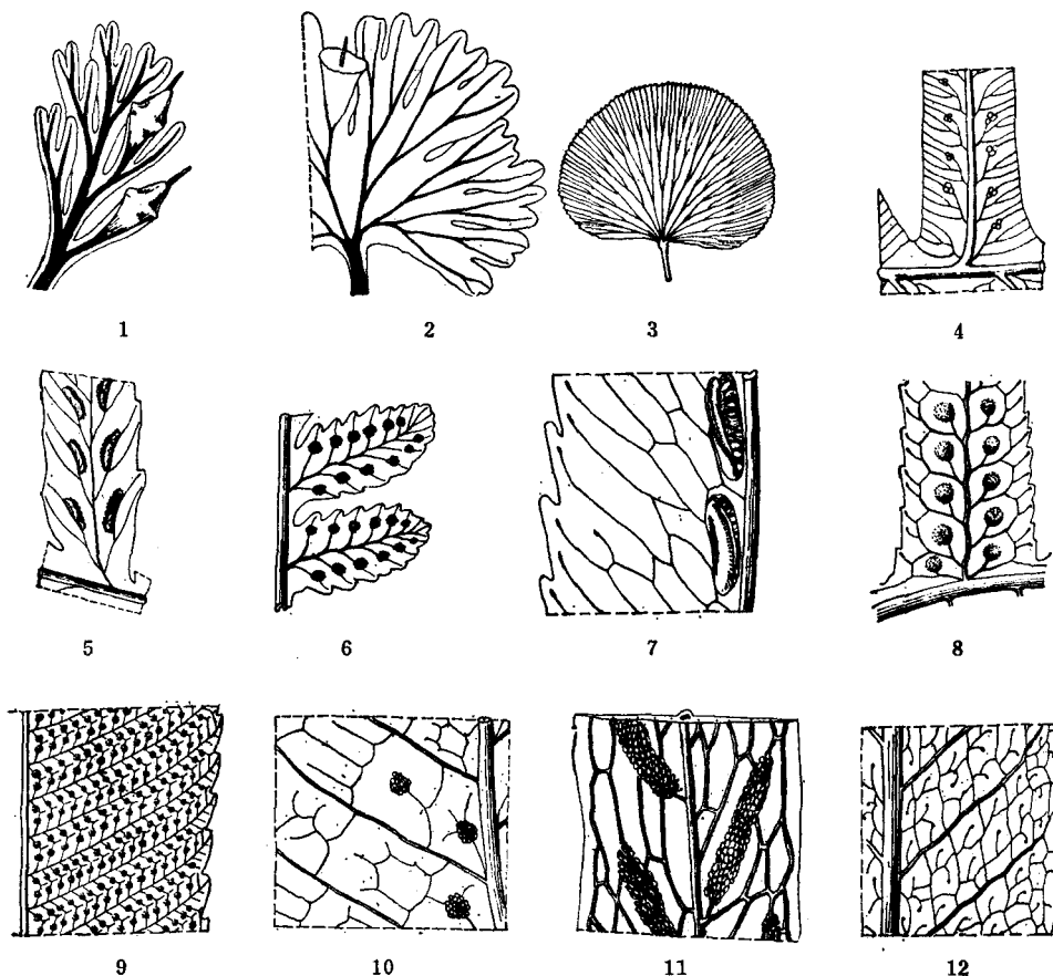
图5 分离型1—6; 中间型7—8; 网结型9—12。
