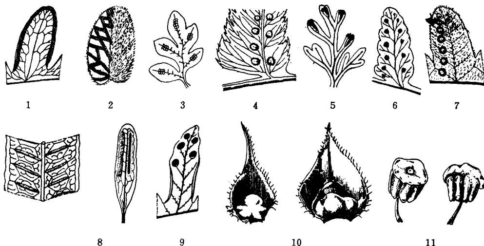
图 6 孢子囊
