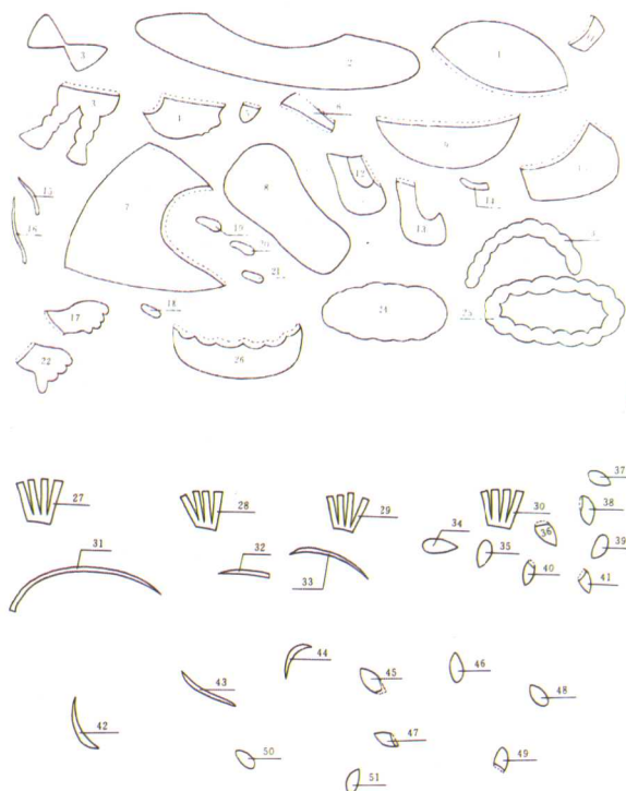
零件图
