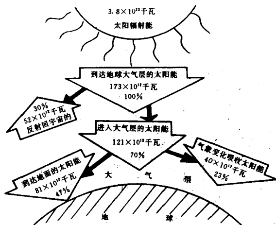
图 2 辐射到地球的太阳能
