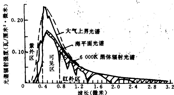
图 3 太阳辐射光谱
