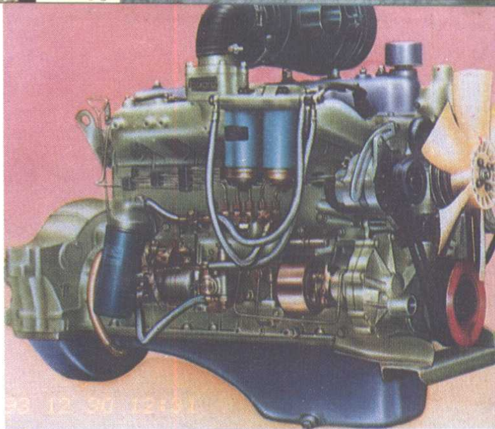
南充内燃机厂生产的 N6102Q 型 柴油机
