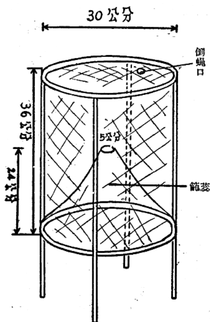
圖4 捕蝇籠。
