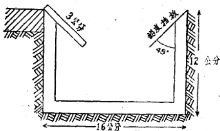
圖 3 捕蛆溝剖面。
