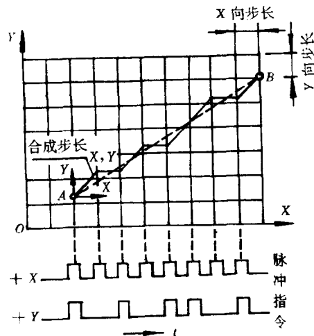
图 1-8 用折线近似逼近直线
