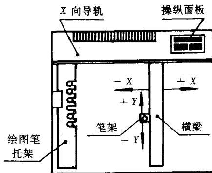
图 1-6 平台式绘图机的结构
