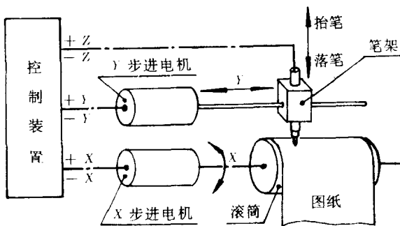
图 1-5 滚筒式绘图机的结构及工作原理
