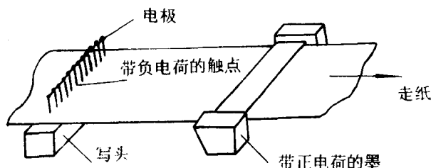
图 1-9 静电式绘图机的结构
