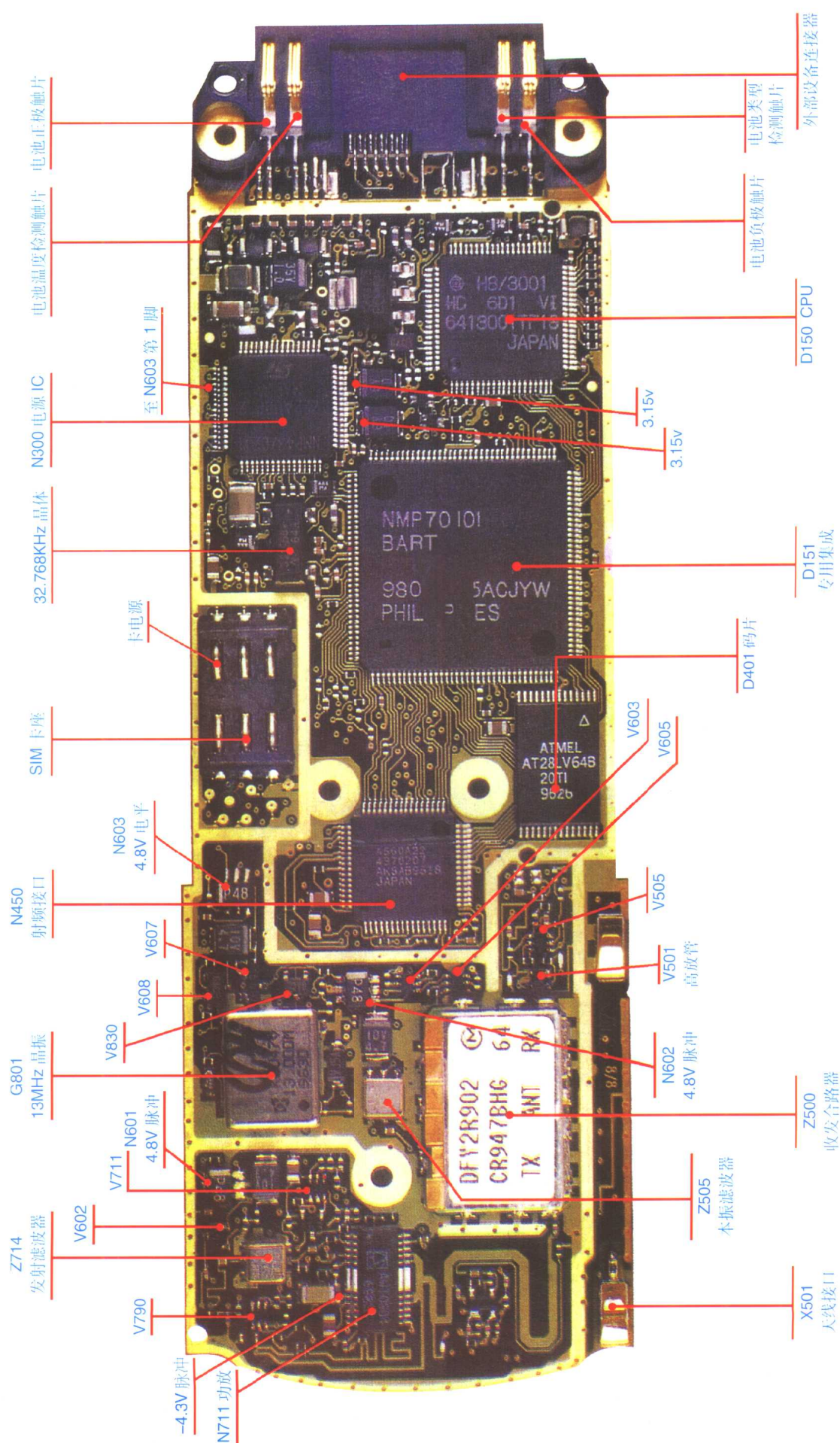
诺基亚 8110 手机主板图二
