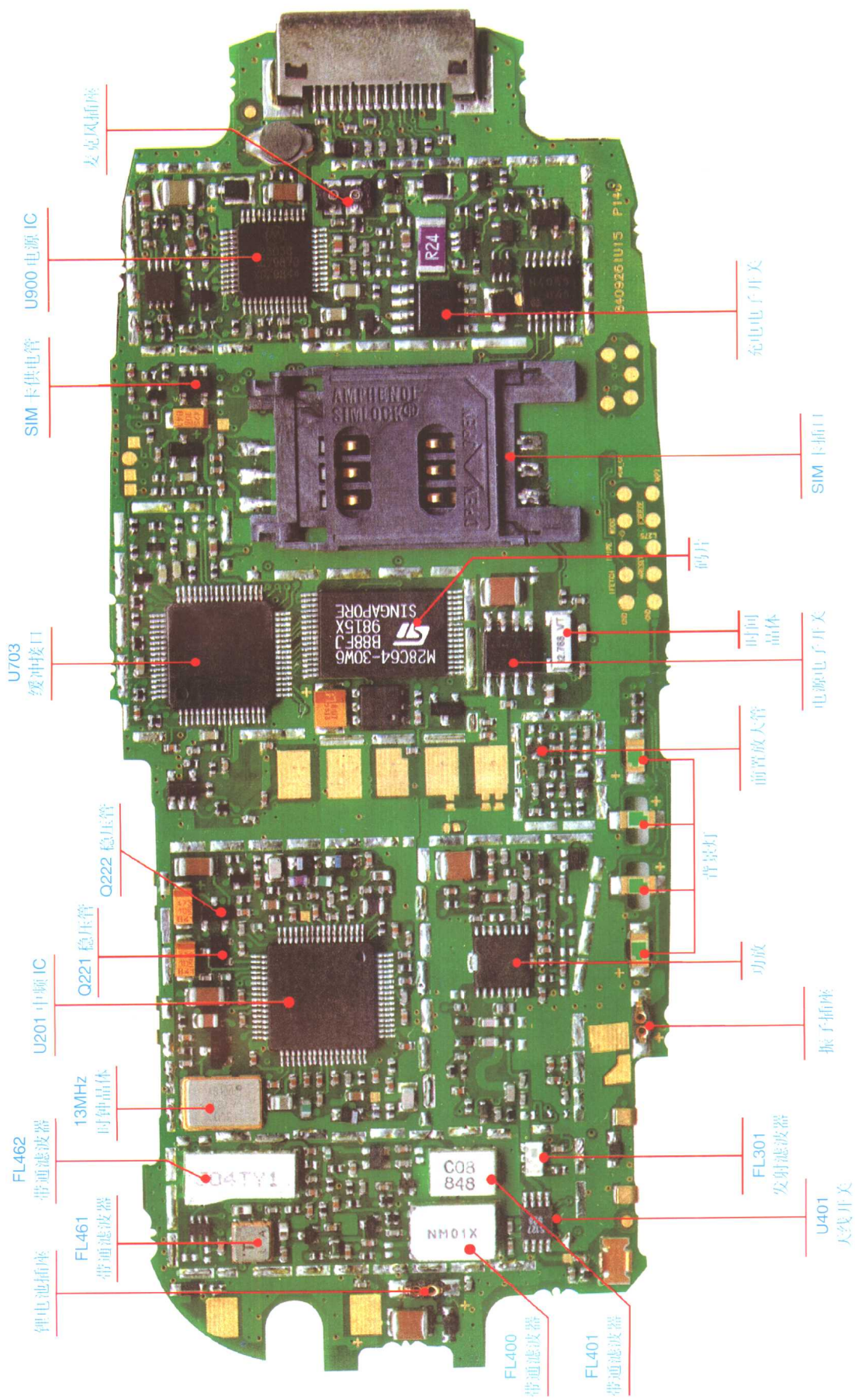
摩托罗拉 cd928 双频手机主板图—
