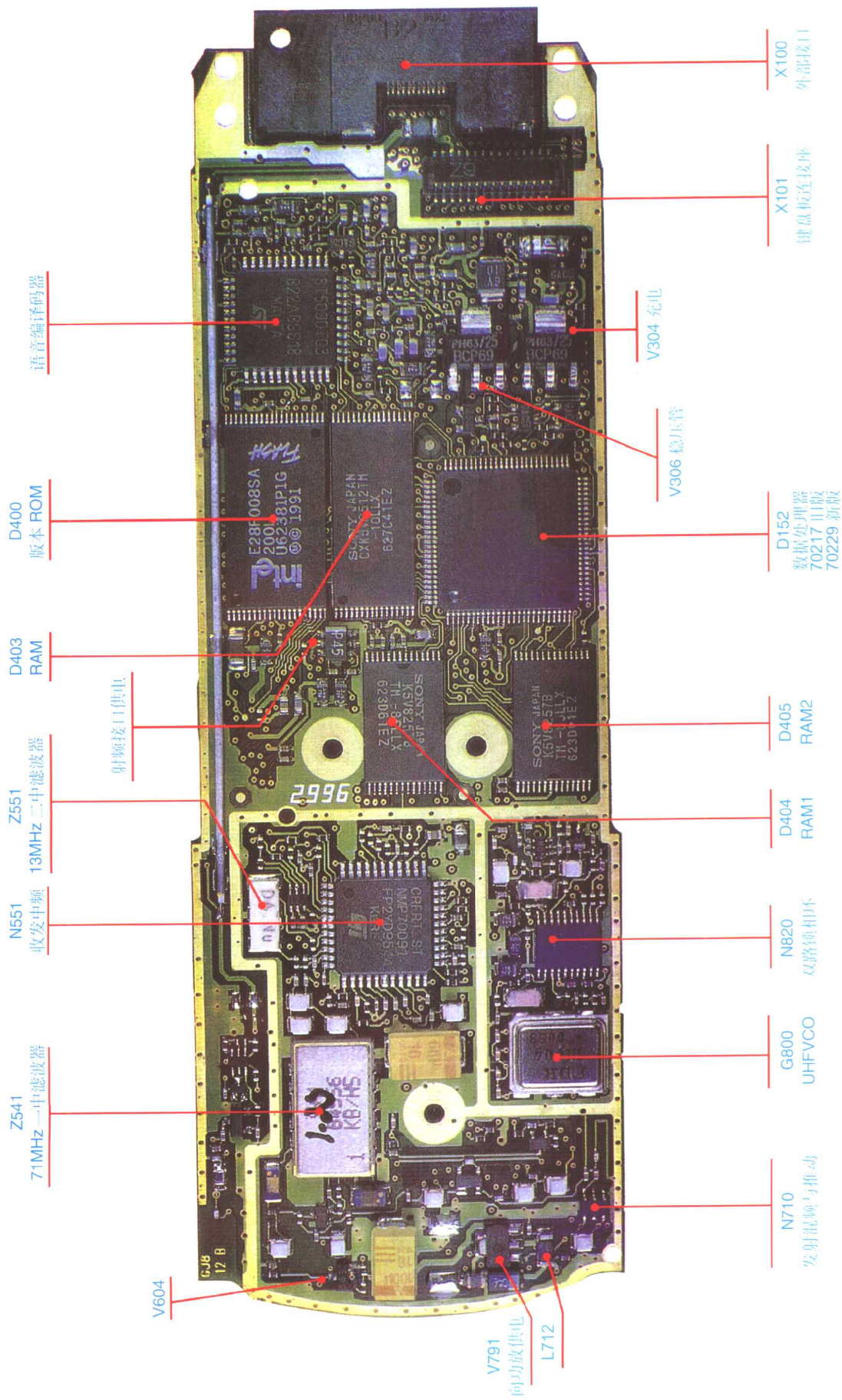
诺基亚 8110 手机主板图一
