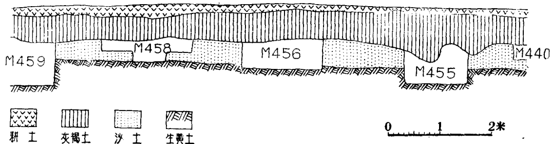
图三 T411 地层剖面图
