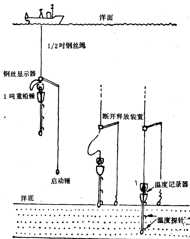
图 4 海洋测温装置原理示意图
