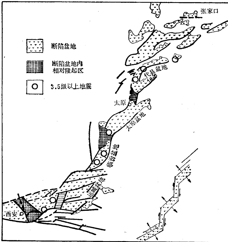
图 2 山西地堑带断陷盆地 (据张文佑等, 1975)
