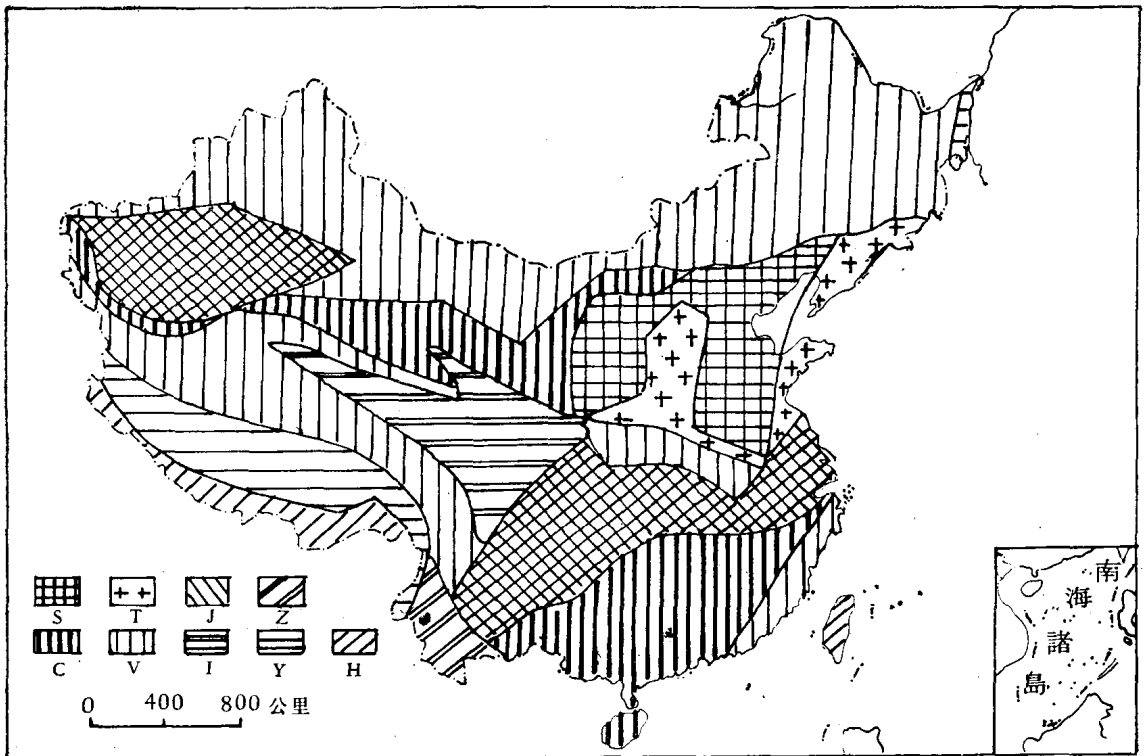
图 1 中国大地构造轮廓
