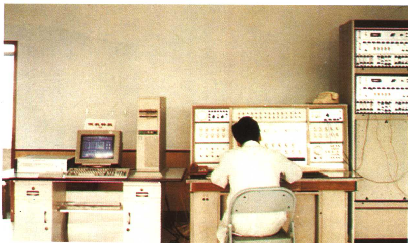
△气象通信监控系统
