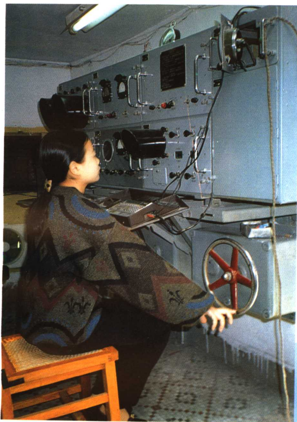
△701 雷达进行高空气象观测
