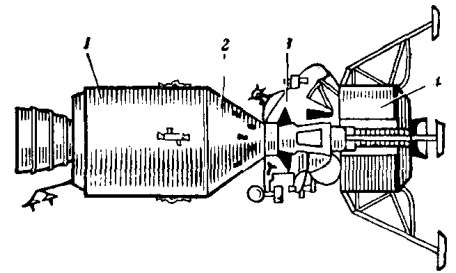
1—宇宙飞船的主要部分; 2—宇航员隔舱; 3—登月舱起飞级; 4—登月舱着陆级
