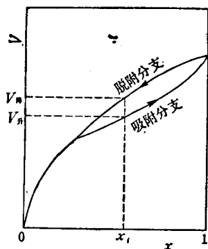
图 1.2 吸附回线
