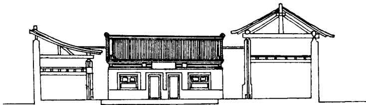
典型的山西民居院落剖面圖
