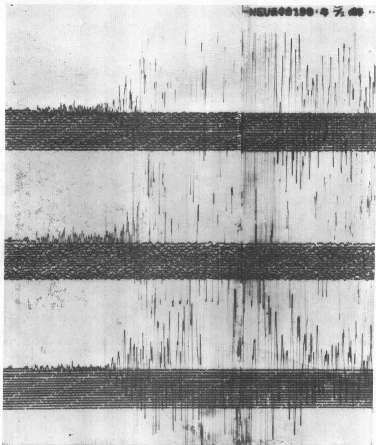
1966年3月22日邢台7.2级地震长春地震台基式地震仪记录图。
