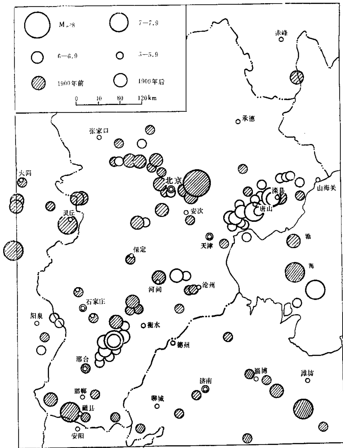
河北省破坏性地震震中分布图。
