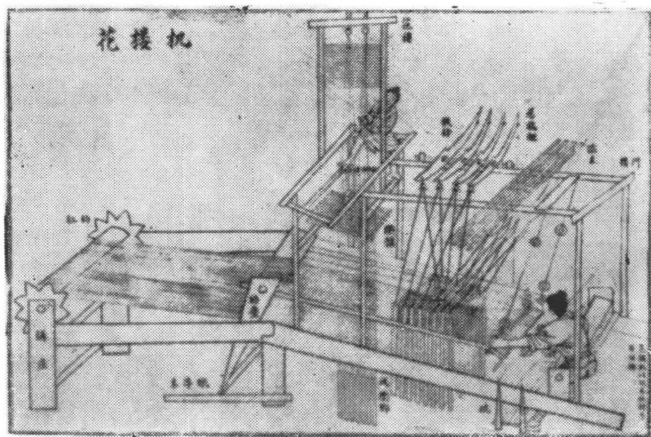
花 楼 机
