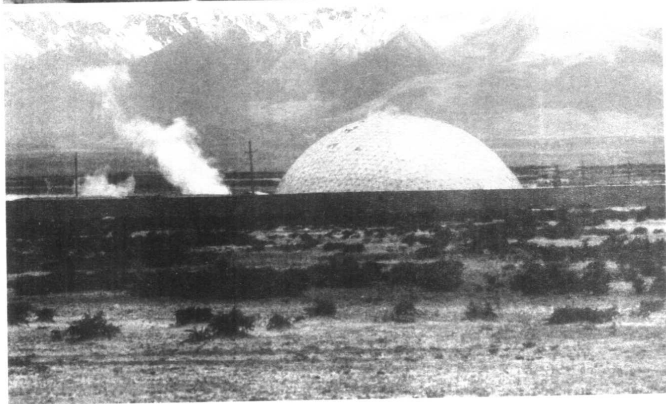
西藏羊八井地热站是我国首次建设的工业性地热试验电站。
