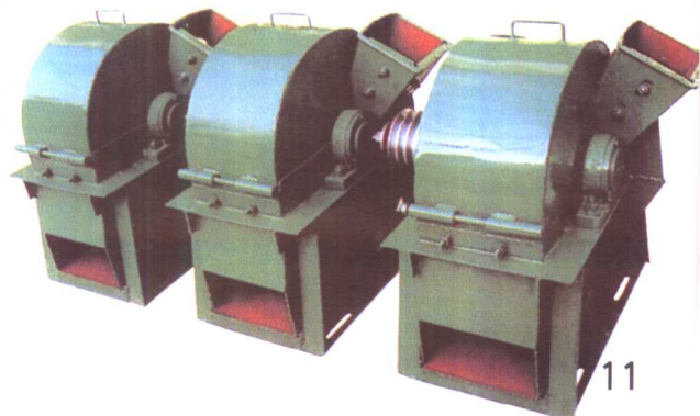
枝桠粉碎机
