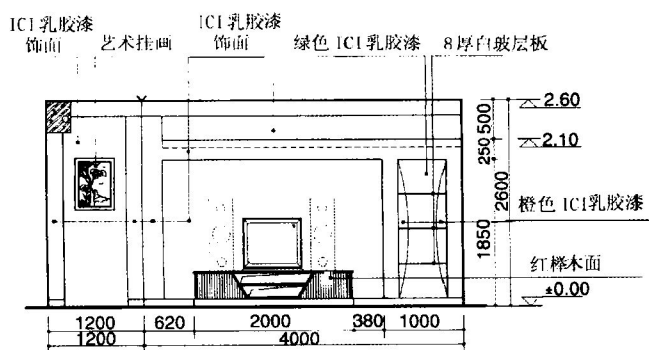
客厅 A 立面图
