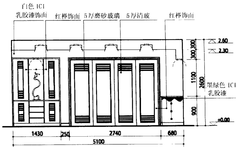
餐厅 C 立面图
