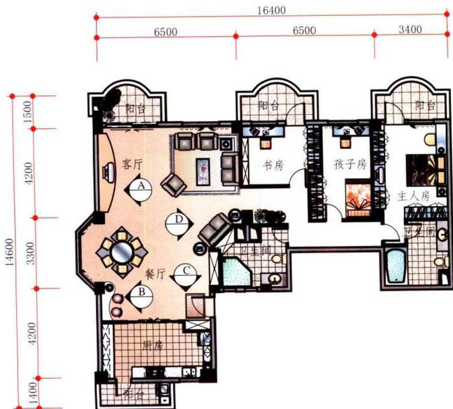
平面布置图 scale 1:180
