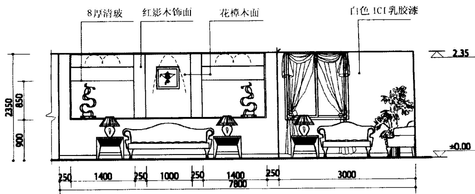
客厅 B 立面图
