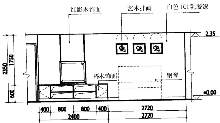
客厅 B 立面图
