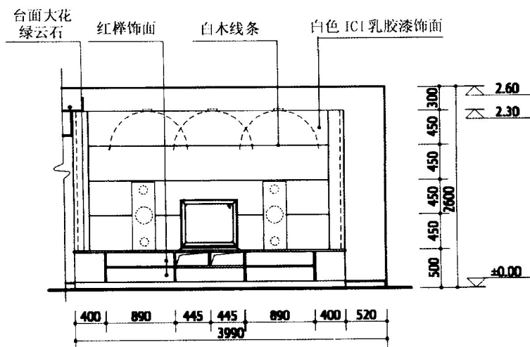
客厅 A 立面图
