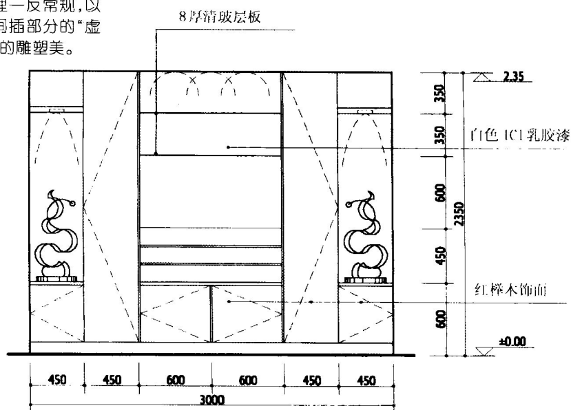
书房 D 立面图
