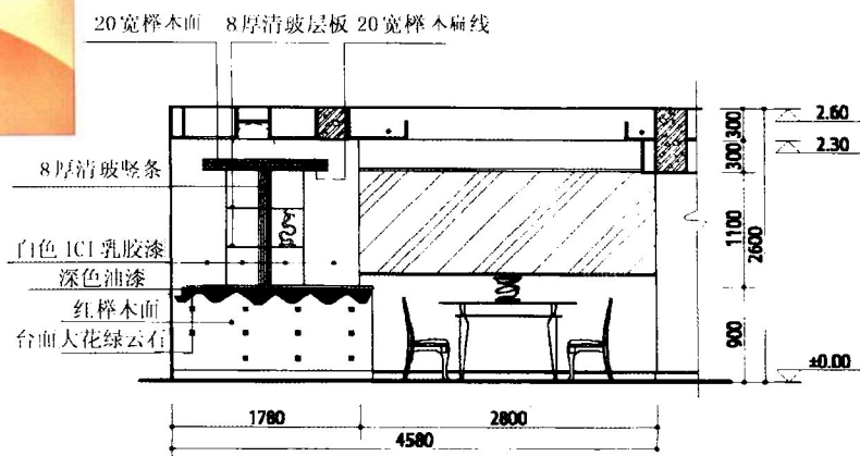
餐厅 B 立面图
