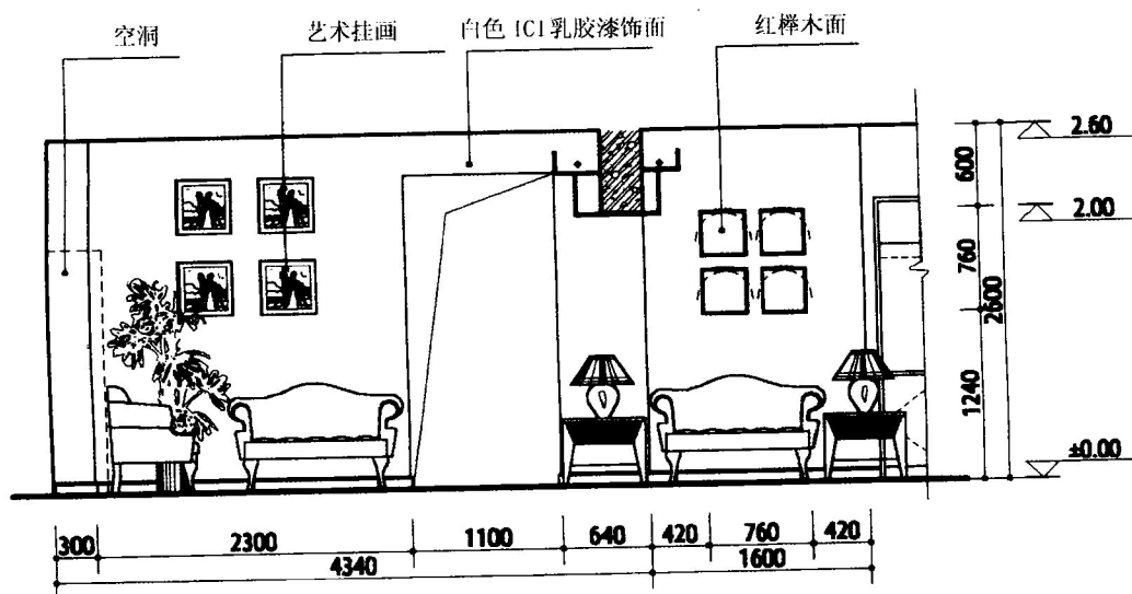
客厅 D 立面图
