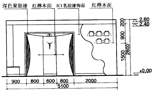
客厅 B 立面图
