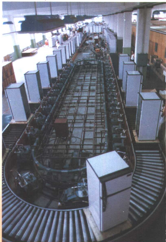
贵州风华电冰箱厂流水生产线车间。 周浩荣 摄
