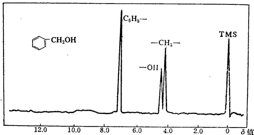
图 12-4 苄醇在 \text{CCl}_4 中的 NMR 图
