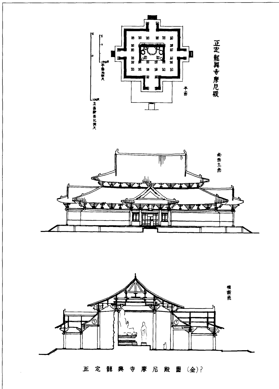
第三图 摩尼殿平面、南立面及横剖面
