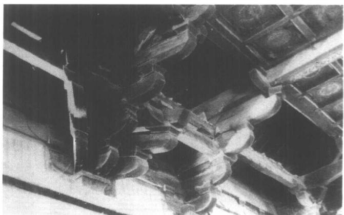
第十图 隆兴寺摩尼殿殿身下檐柱头铺作及补间铺作后尾
