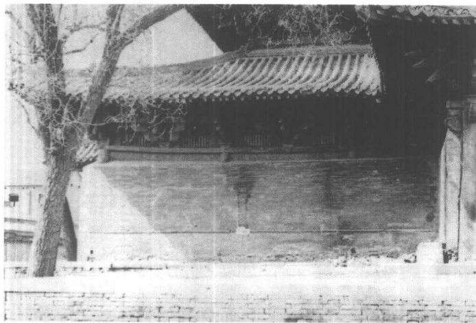
第七图 隆兴寺摩尼殿角柱之生起
