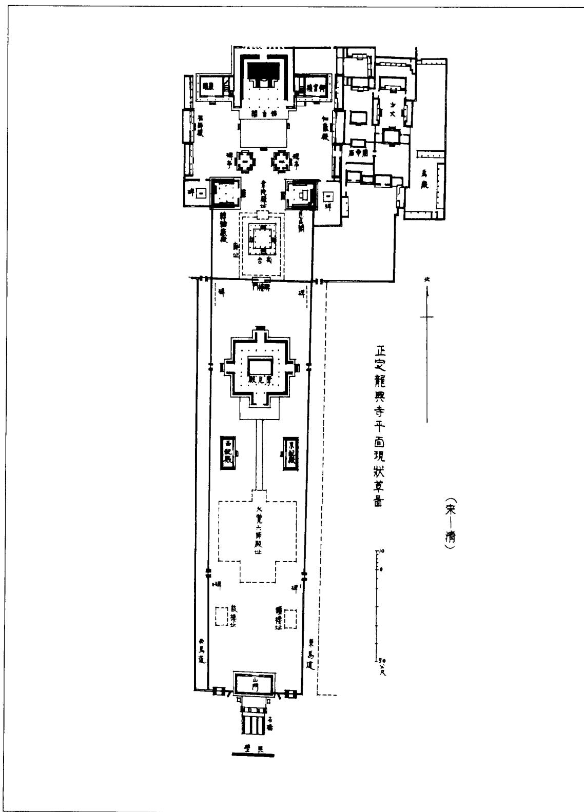
第一图 隆兴寺(龙兴寺)平面现状草图
